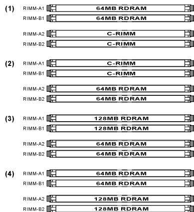
Figure 2-5. Exemple de configurations des modules mémoire
