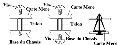
Figure 2-2. La manière de fixer la Carte Mère
