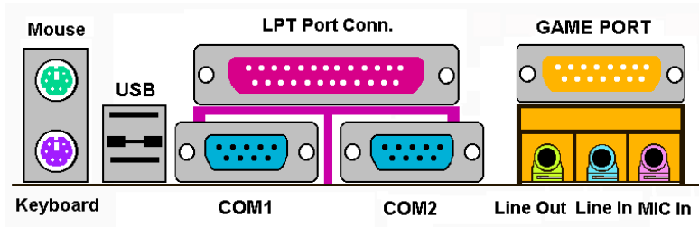
Figure 2-11. Disposition des connecteurs arrière de la SE6
