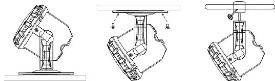
Auf einer horizontalen Oberfläche befestigt | Befestigung an der Decke oder Wand | Befestigung an einem Träger (zB. ALU Truss)
