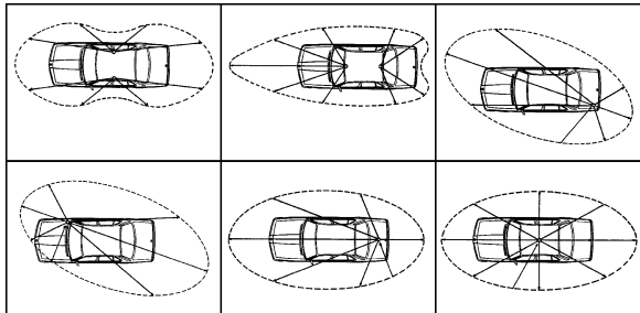
ANTENNEN-DIAGRAMM
