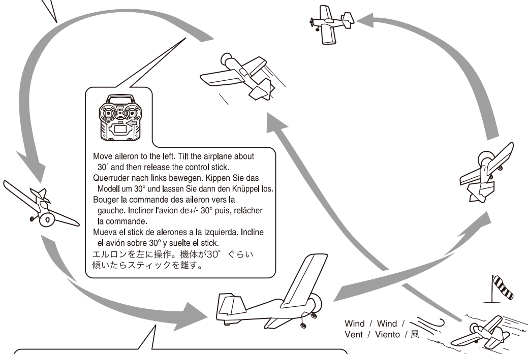
Mode 2
