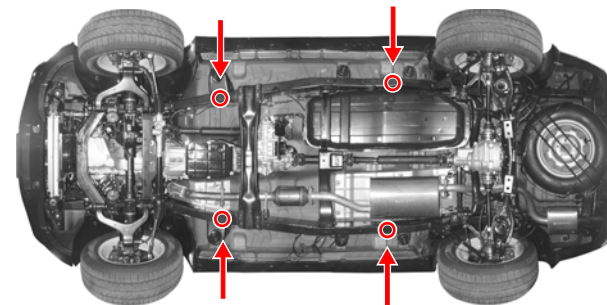
<Points de mise sur cric >
