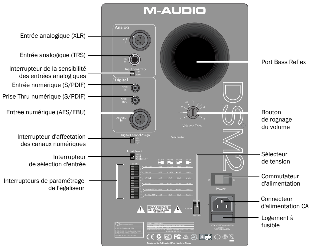
Figure 1. Panneau arrière du haut-parleur DSM2
