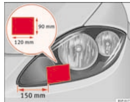
Fig. 130 Phare gauche ▶
