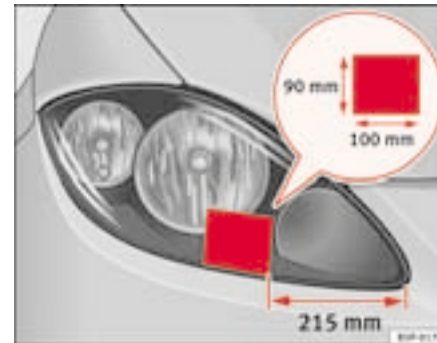
Fig. 129 Phare droit
