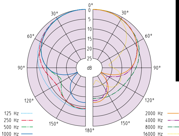
Directivité
