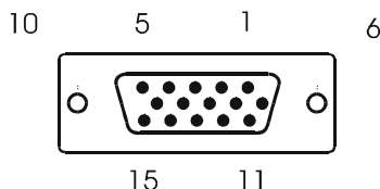
Connecteur D-Sub Mini Pin 15
