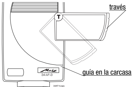
Grabado 7: Montaje/desmontaje de difusores
