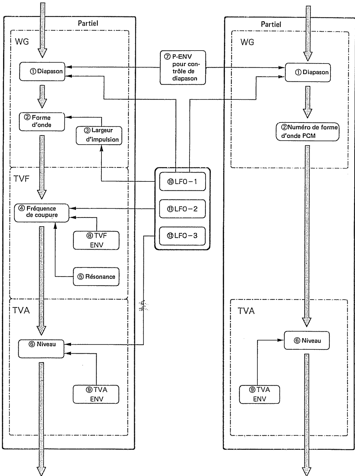
Générateur de son PCM
