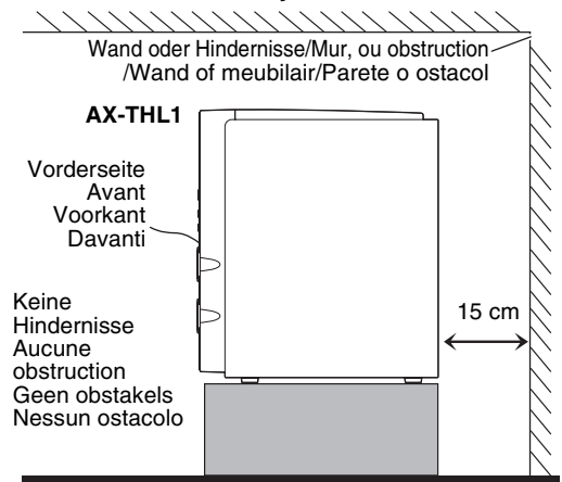
Seitenansicht/Côté/Zijaanzicht/Vista laterale
