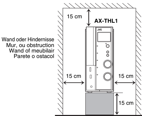
Vorderansicht/Face/Vooraanzicht/Vista frontale
