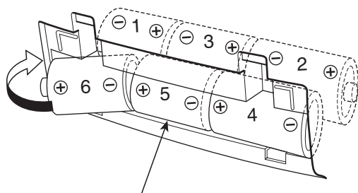
Piles de taille R20 (SUM-1)/D (13D)
