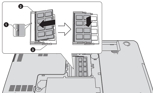
Illustration 4-11 Pose du module mémoire
