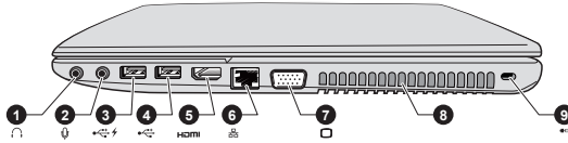
Illustration 3-3 Ordinateur vu de droite
