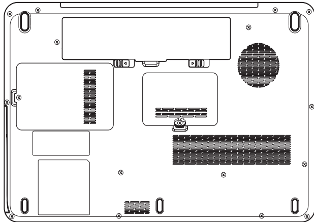
Illustration 8-3 Retrait du capot du module mémoire
