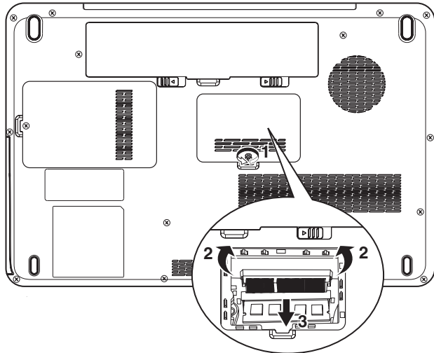
Illustration 8-2 Retrait du couvercle du module mémoire
