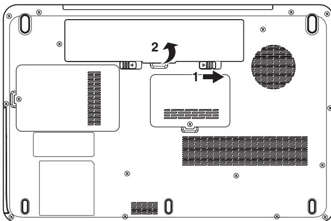
Illustration 6-2 Retrait de la batterie (2)
