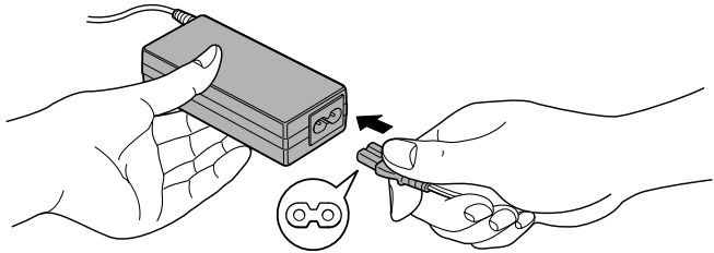
Illustration 3-1 Connexion du cordon d'alimentation à l'adaptateur (prise à 2 fiches)
