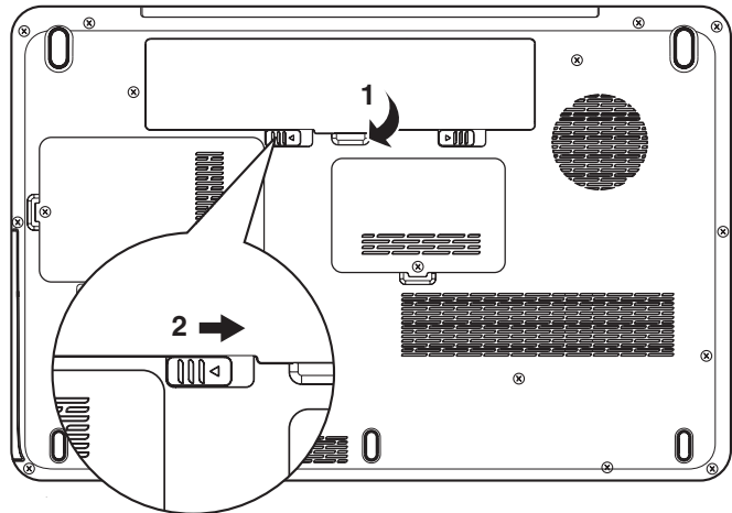
Illustration 6-3 Sécurisation de la batterie
