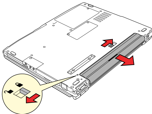
Retrait de la batterie
