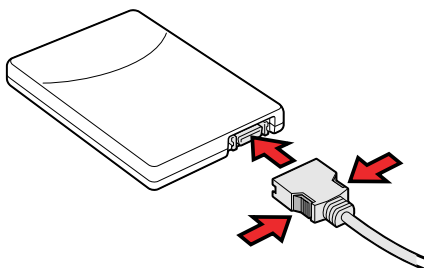
Connexion du câble au lecteur de disquettes
