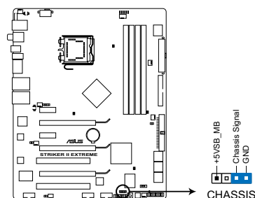
Connecteur du détecteur d'intrusion châssis de la Striker II Extreme/Striker II NSE
