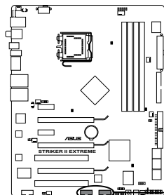
Connecteurs USB 2.0 de la Striker II Extreme/Striker II NSE
