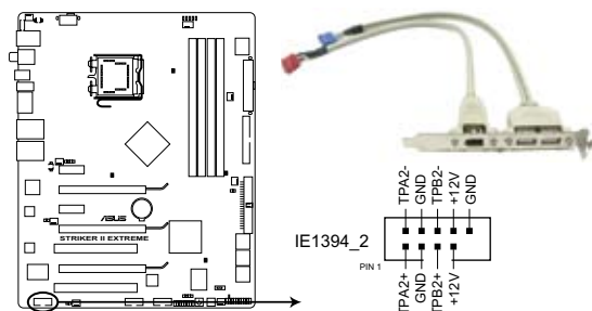
Connecteur 1394a de la Striker II Extreme/Striker II NSE
