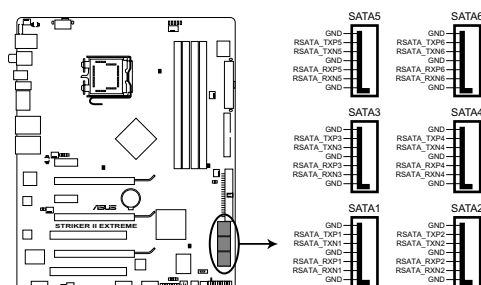
Connecteurs SATA de la Striker II Extreme/Striker II NSE
