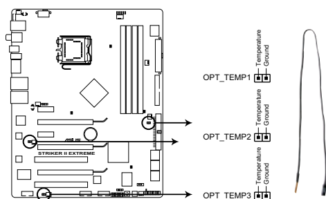
Connecteur de câble de détection thermique de la Striker II Extreme/Striker II NSE
