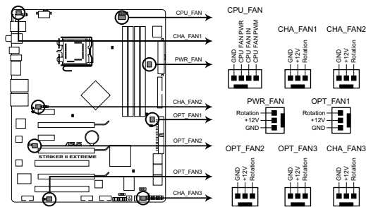
Connecteurs de ventilation de la Striker II Extreme/Striker II NSE
