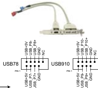
Connecteurs USB 2.0 de la Striker II Extreme/Striker II NSE
