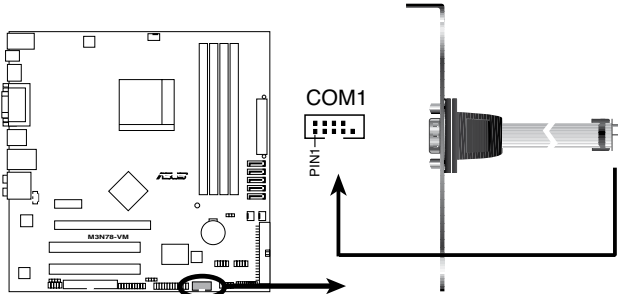
Connecteur port série de la M3N78-VM
