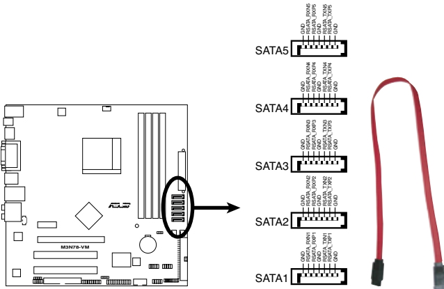
Connecteurs SATA de la M3N78-VM
