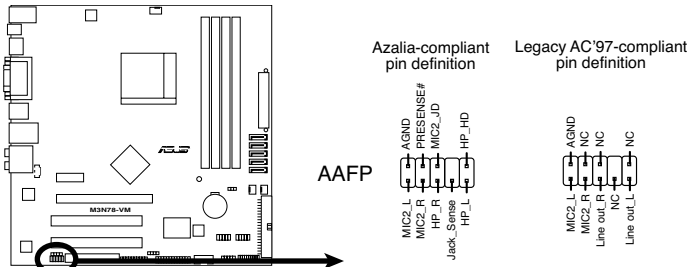
Connecteur audio en façade de la M3N78
