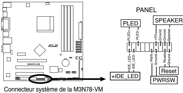
Connecteur système de la M3N78-VM
