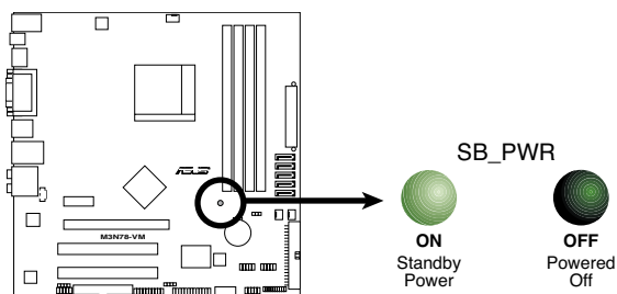
LED embarquée de la M3N78-VM
