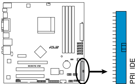
Connecteur IDE de la M3N78-VM
