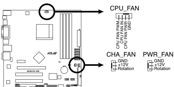
Connecteurs de ventilation de la M3N78-VM
