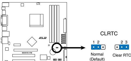
Clear RTC RAM de la M3N78-VM
