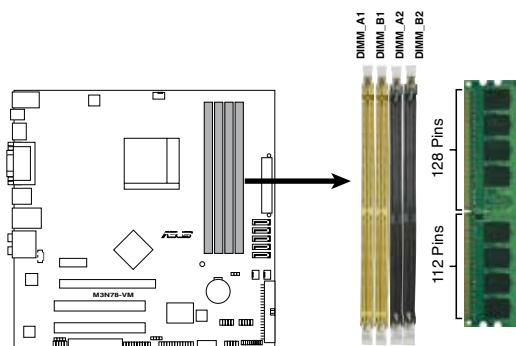
Sockets DIMM DDR2 de la M3N78-VM
