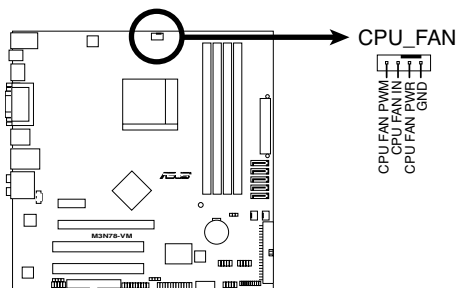
Connecteur du ventilateur du CPU de la M3N78-VM
