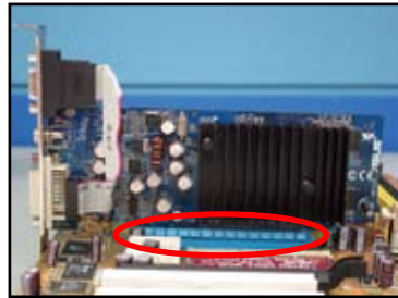
Carte PCIE x16
