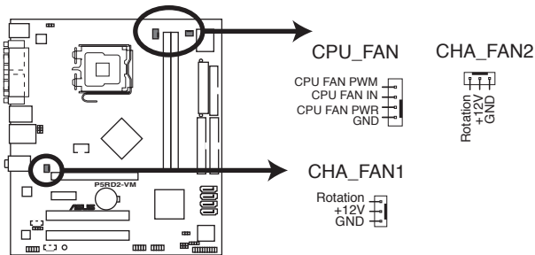
Connecteurs de ventilation de la P5RD2-VM
