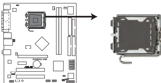
Socket 775 du CPU de la P5RD2-VM
