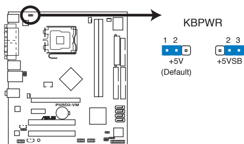
Paramètres d'alimentation du clavier de la P5RD2-VM
