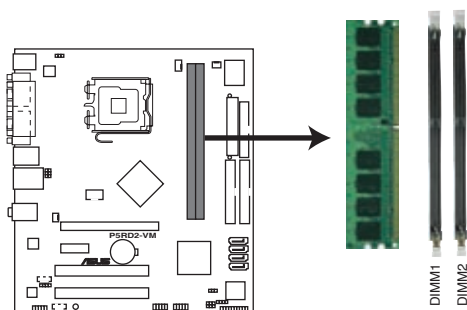
Sockets DIMM de la P5RD2-VM
