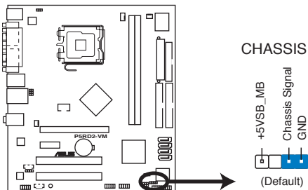
Connecteur chassis intrusion de la P5RD2-VM
