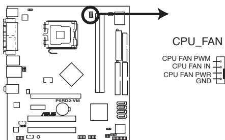
CPU_FAN de la P5RD2-VM
