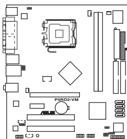
Connecteur pour lecteur de disquettes de la P5RD2-VM
