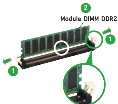
Clip de rétention déverrouillé
