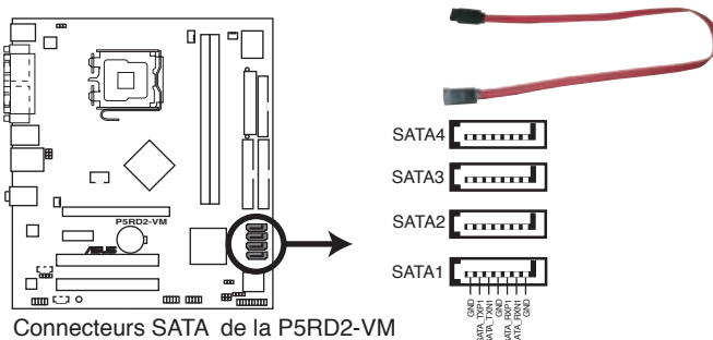
Connecteurs SATA de la P5RD2-VM
