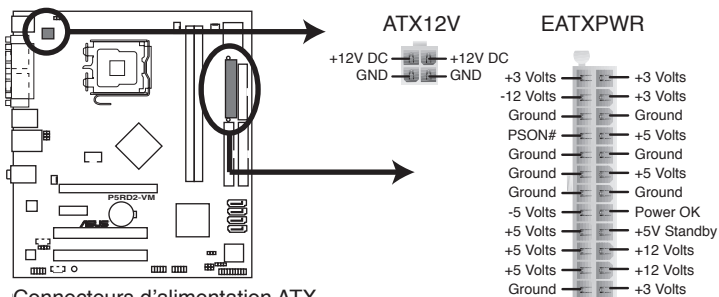
Connecteurs d'alimentation ATX de la P5RD2-VM
