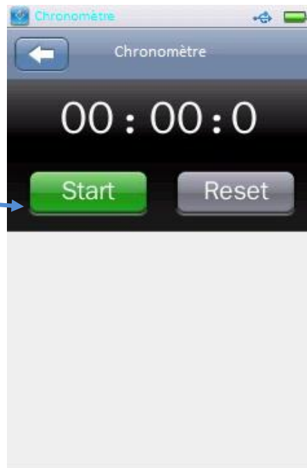
Interface Chronomètre
