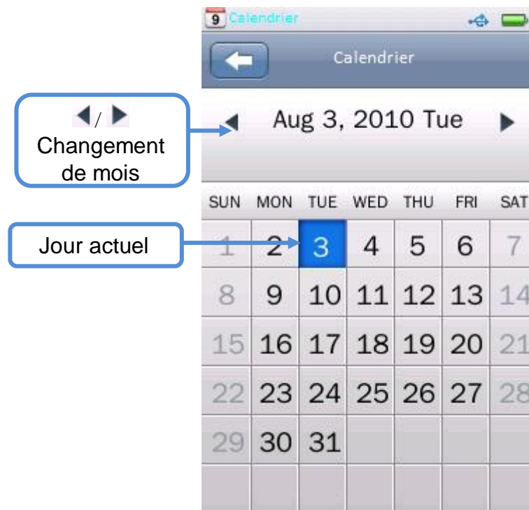
Interface Calendrier
