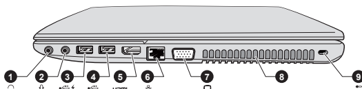
Illustration 2-3 Ordinateur vu de droite
