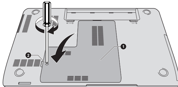
Illustration 3-14 Retrait du capot du module mémoire
