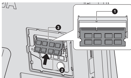
Illustration 4-9 Pose du module mémoire
