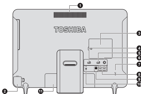
Illustration 3-4 Vue arrière de l'ordinateur
