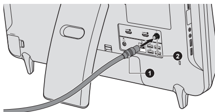
Illustration 4-14 Connexion du câble coaxial
