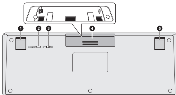
Illustration 3-7 Arrière du clavier sans fil
