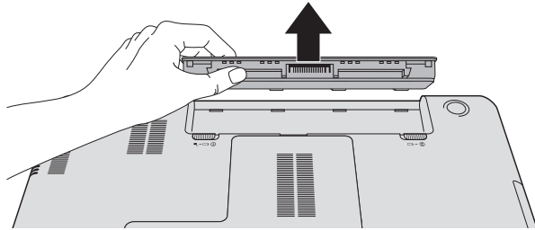
Illustration 4-10 Retrait de la batterie - 2
