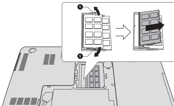
Illustration 4-14 Retrait d'un module mémoire
