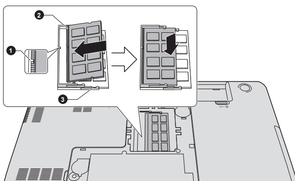
Illustration 4-12 Pose du module mémoire
