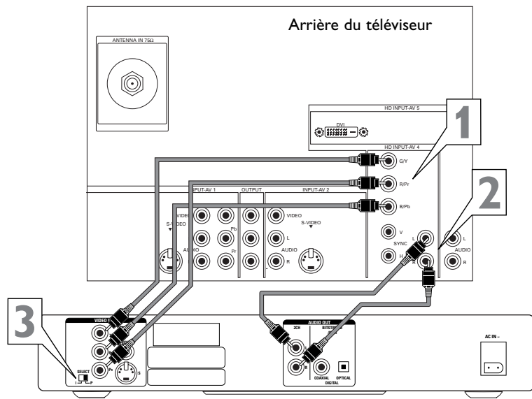
Arrière du lecteur DVD à balayage progressif
