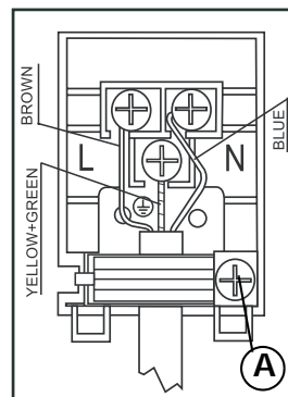
Schéma des branchements électriques
