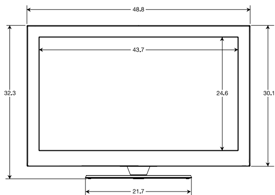
VUE AVANT
