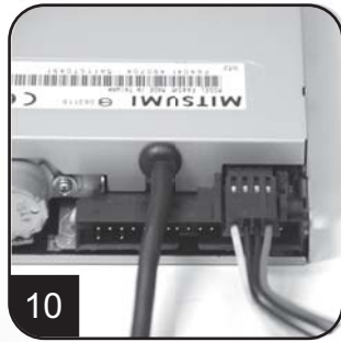
10 작은 4핀 전원케이블은 플로피 드라이브 또는 다른 호환 장치에 연결하십시오
