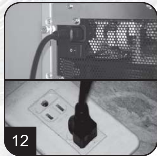
12 파워서플라이에 AC 전원케이블을 연결하십시오. (주의사항: 가급적 연장 소켓을 사용하지 마십시오, 꼭 필요하다면 사용되되, TV나 오디오 같은 고출력의 가전제품과 같은 소켓에 혼용하여 사용하지 마십시오.
