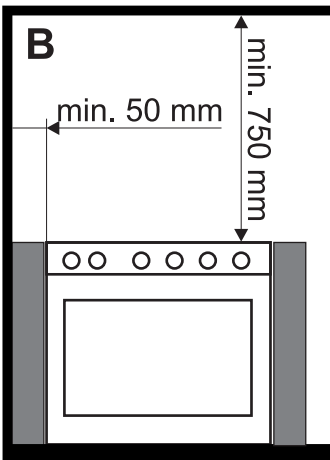
B - Classe 2 sous-classe 1 (Appareil encastré)
