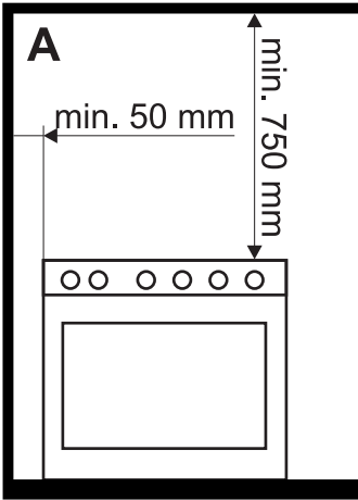
A - Classe 1 (Appareil pour installation libre)
