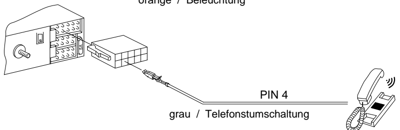
orange / Beleuchtung
