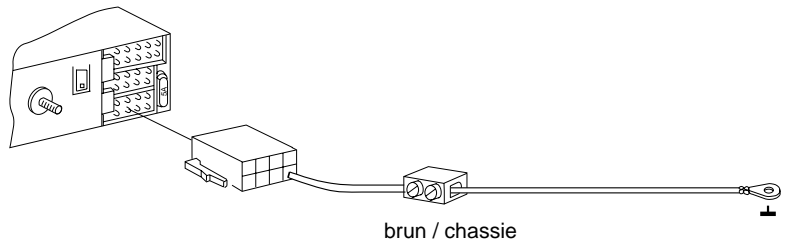
brun / chassie
