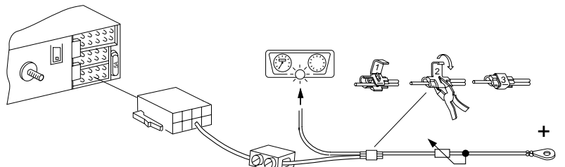
orange / Beleuchtung
