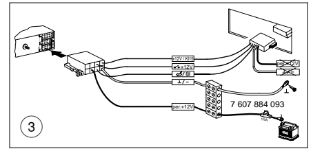
Conexión del autorradio con el cable adaptador y cable de conexión
