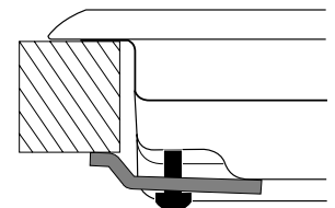
Posizione gancio per top H=30mm
