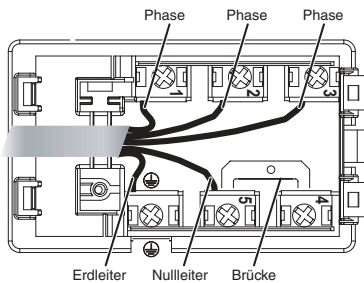
Dreiphasenanschluss 400
