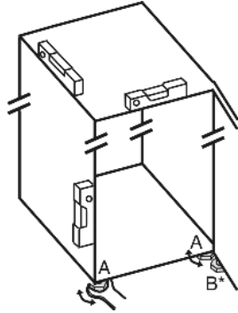
Fig. 4 pour les appareils dotés d'une poignée de porte
