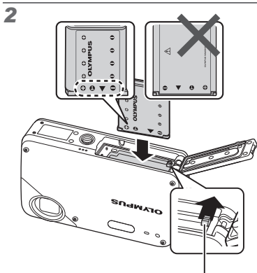
Touche de verrouillage de la batterie
