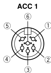
Vue du panneau arrière du TS-450S/690S/850S/950SDX
