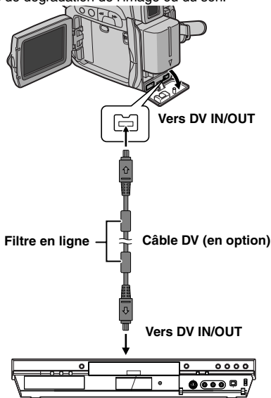
Appareil vidéo équipé d'un connecteur DV
