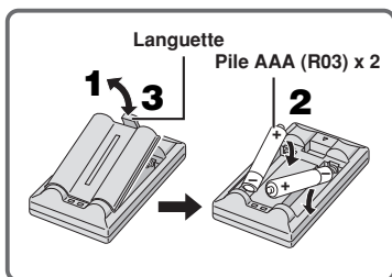
Télécommande RM-V717U
