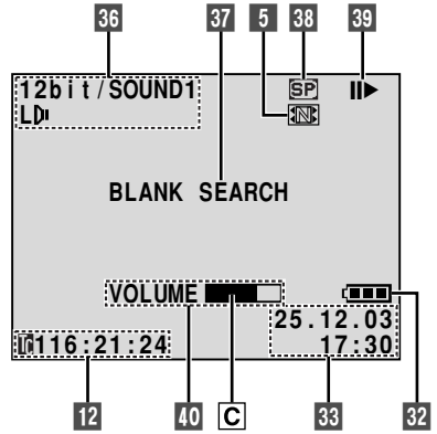
Pendant la lecture sur bande
