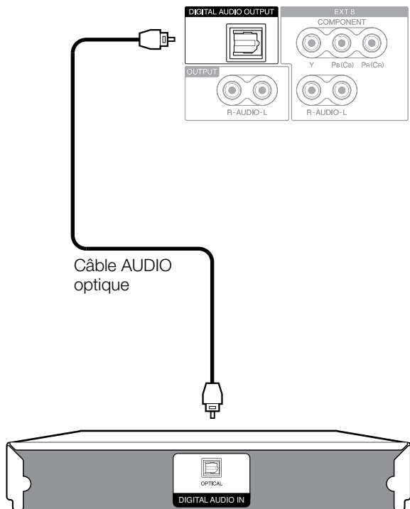
Amplificateur avec entrée audio numérique
