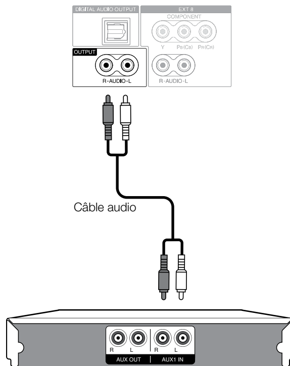
Amplificateur avec entrée audio analogique
