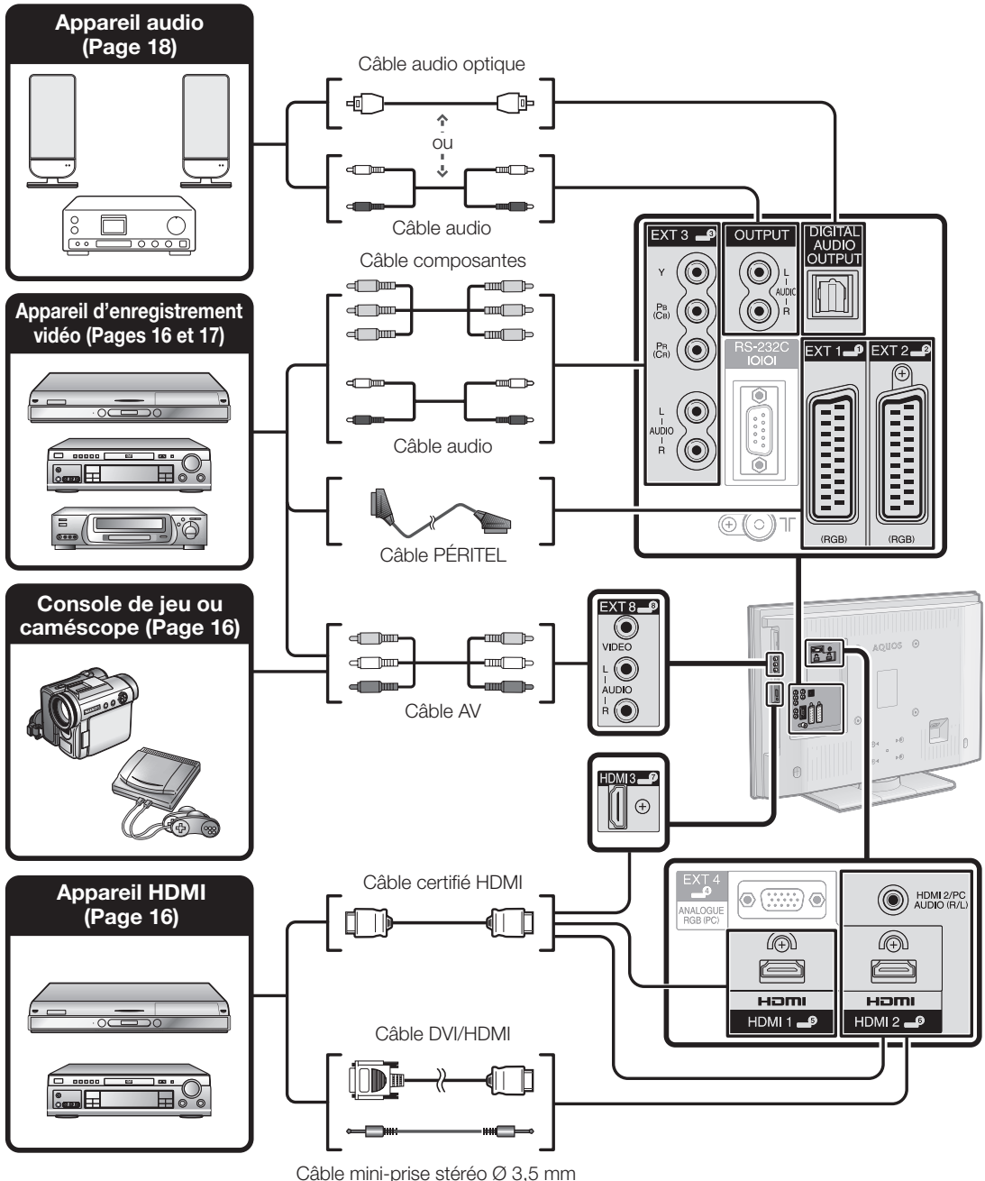
Câble mini-prise stéréo Ø 3,5 mm
