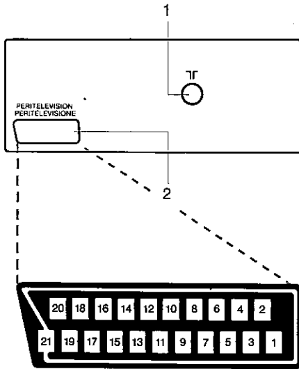
21-polige Euro-SCART
