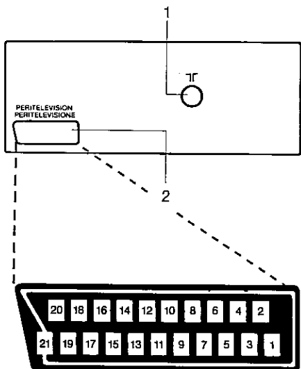
Prise péritel
