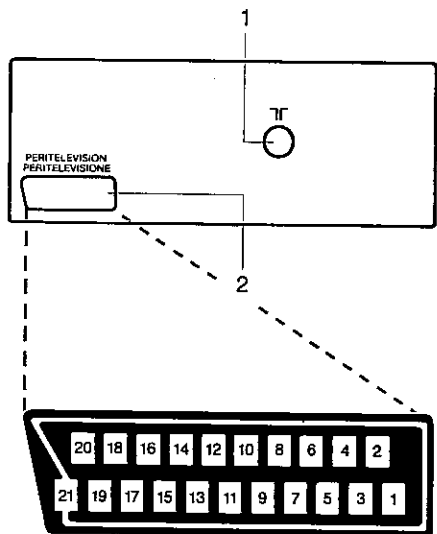
21-pol. Euro-SCART-Buchse
