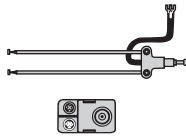
Antenne droite (dipôle) avec ruban d'alimentation Convertisseur d'impédance 300-75 (Seulement pour 14J1-GF/14J1-SF)
