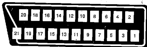
Péritel à 21 broches
