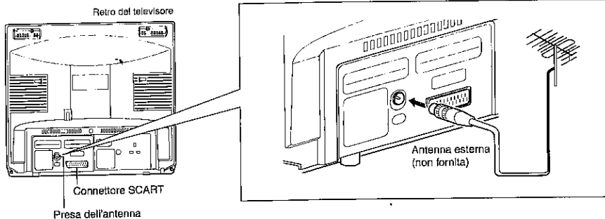
Cavo coassiale da 75 ohm (cavo tondo)
