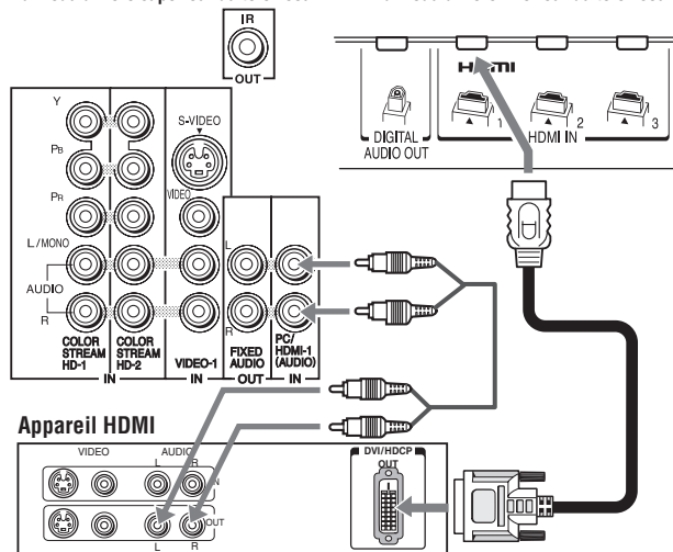
Panneau arrière supérieur du téléviseur
