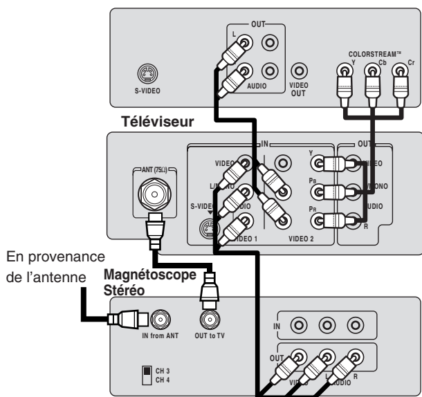
Lecteur DVD avec ColorStream®
