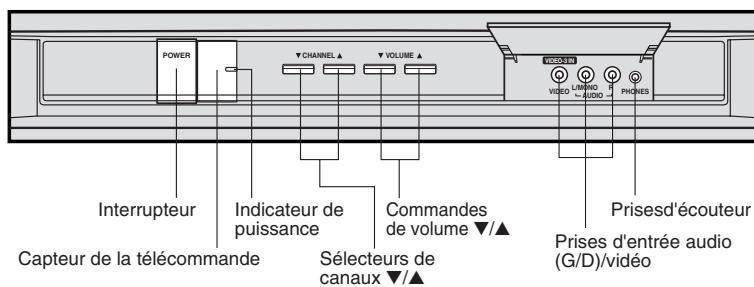
Panneau avant du téléviseur
