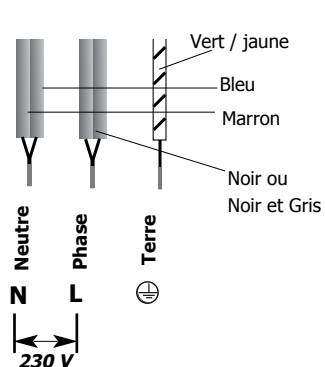
fusible : 32 ampères
