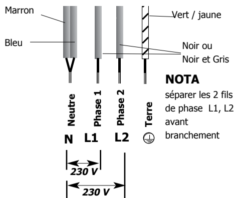
fusible : 16 ampères
