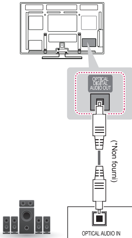
Système audio numérique
