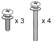
M5 x 16 M4 x 30 Vis de montage (Voir la page13, Voir la page14)
