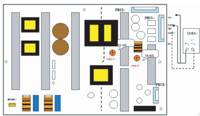
(Illustrazione. 4) Diagramma di connessione per regolazione/messa a punto e misura fonti di energia.
