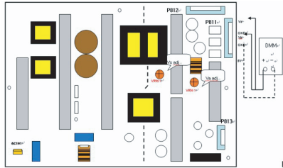
(Illustrazione. 3) Diagramma di connessione per regolazione/messa a punto e misura fonti di energia.
